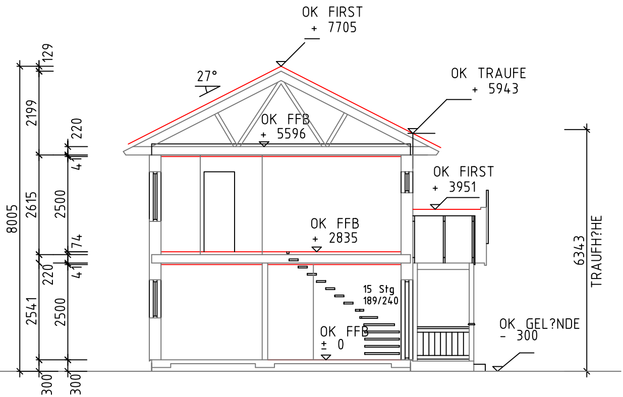
SCHNITT A-A
